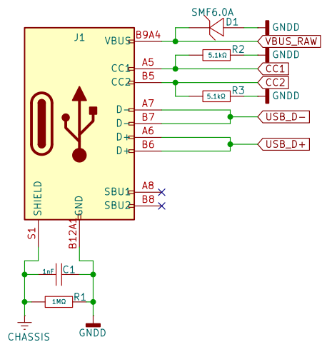
ESD/TVS protection
