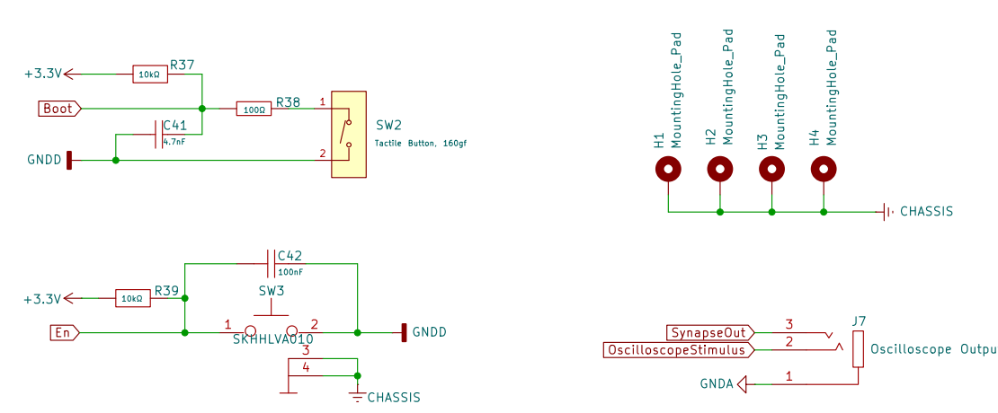
ESP32 Buttons
